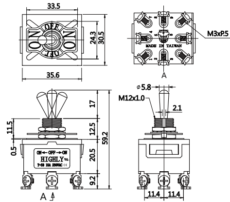
T-32BS / T-33BS 3PDT
