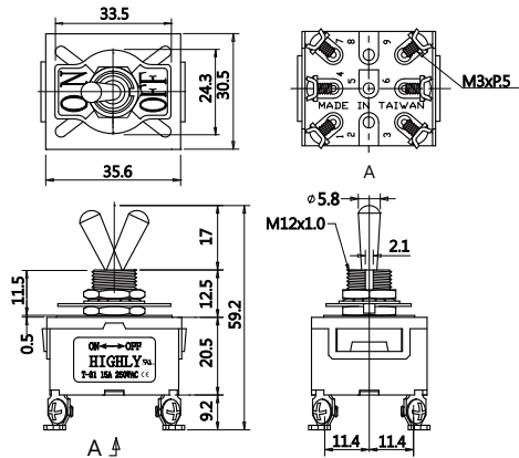
Function Type T-31BS 3PST
