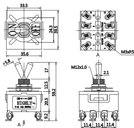
Function Type T-41BS 4PST
