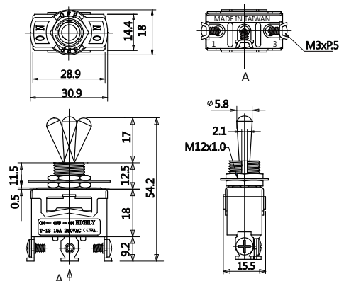
T-12BS / T-13BS SPDT
