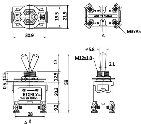
Function Type T-21BS DPST
